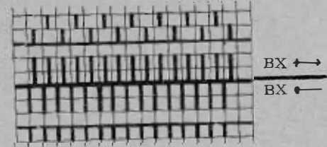
Schéma jacquard
