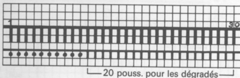
Disposition des aiguilles et des poussoirs pour le col
